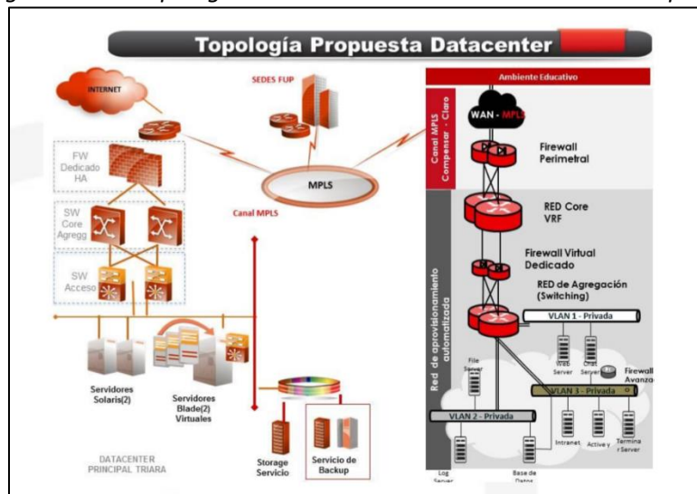
Figura 68 68. Topología en Datacenter de los servicios de UCompensar
