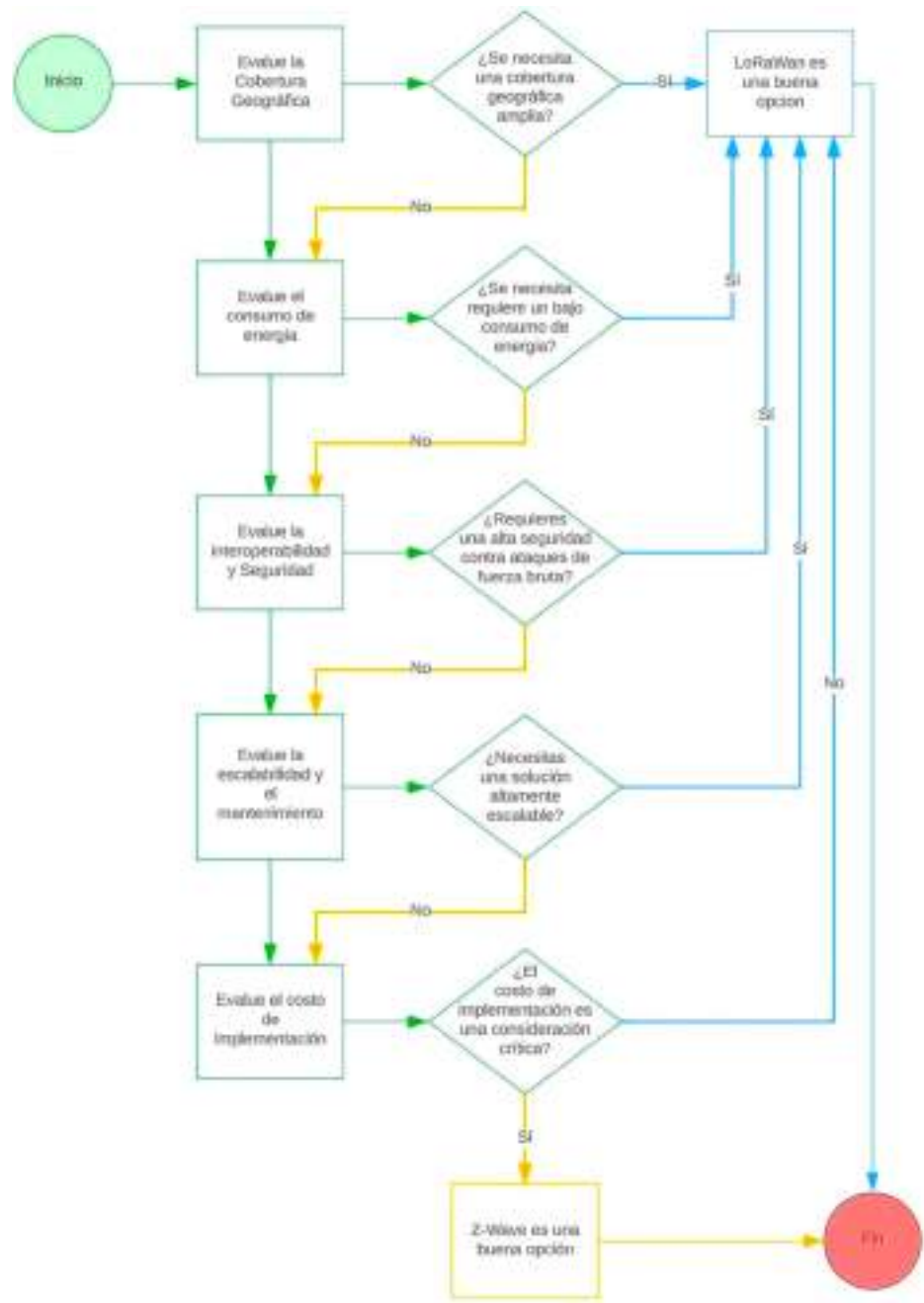
Figura 15. Diagrama de flujo selección de protocolo
